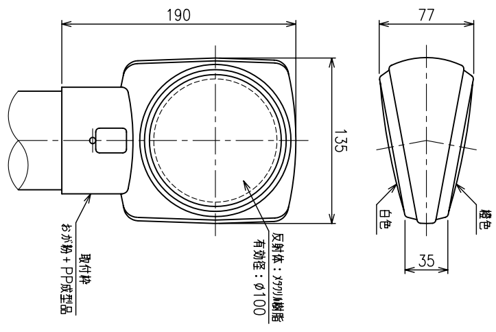
反射部 詳細図 S=1:3
